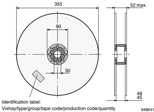
Fig. 24 - Reel
