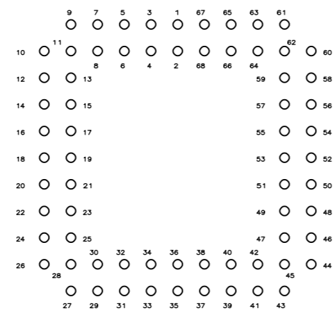
68 POS.
